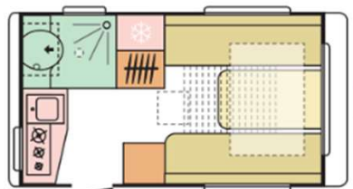
361 LH Posti letto 2/3 Peso da Kg 1.000 Lungh. Int 3.61 m Lungh. Est 5.22 m Largh. 2.19 m
